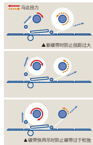
双碳带电机自动控制示意图▶
